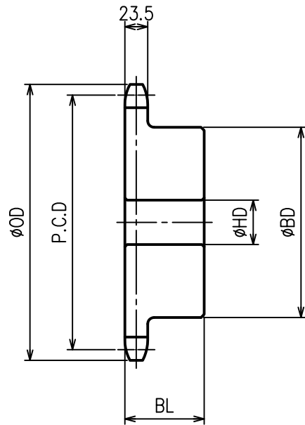
120 スプロケット - B形 -
