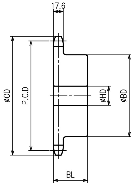
100 スプロケット - B形 -
