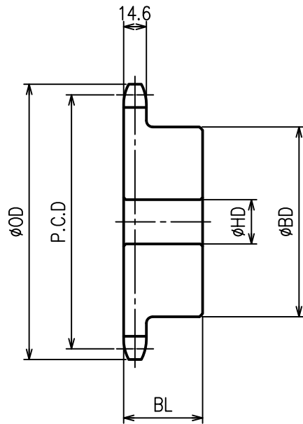
80 スプロケット - B形 -
