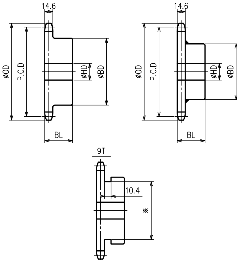
80 スプロケット - 新B・BW形 -
