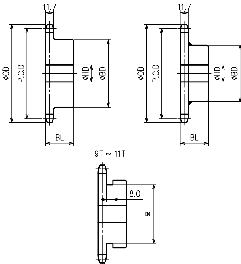
60 スプロケット - 新B・BW形 -
