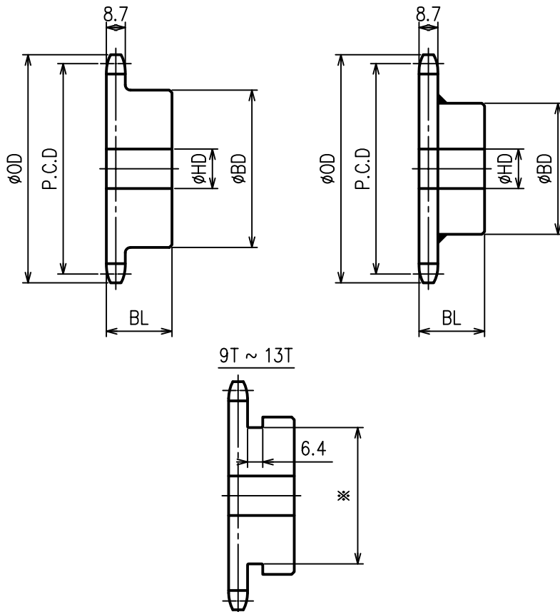
50 スプロケット - 新B・BW形 -
