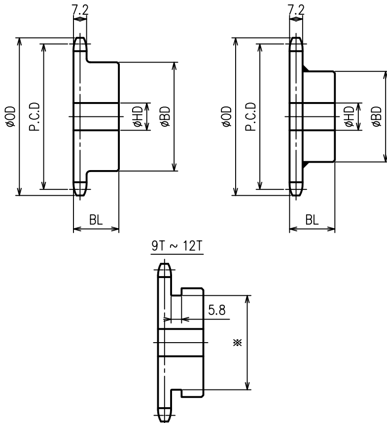
40 スプロケット - 新B・BW形 -
